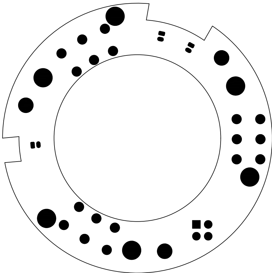
Защитная паяльная маска рисунок 12
